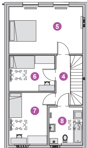
Rzut poddasza
